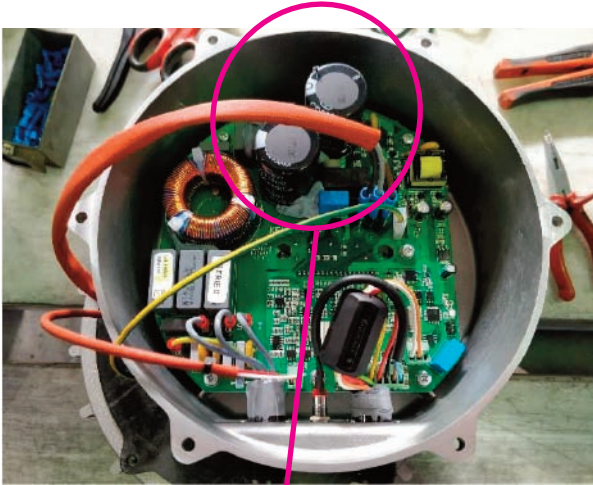
Condensadores electrolíticos
