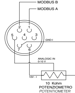
DETTAGLIO CONNESSIONI
